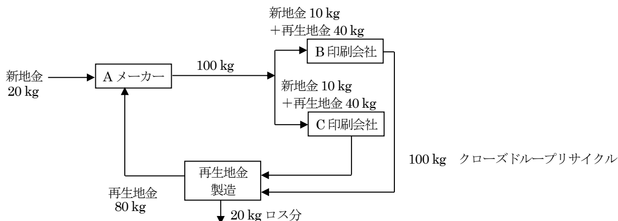
図5 クローズドループリサイクルの場合(再生地金製造時20%ロスの場合)
