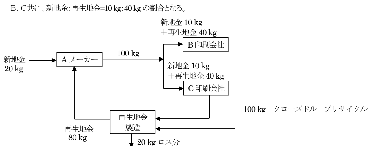
図5 クローズドループリサイクルの場合(再生地金製造時20%ロスの場合)
