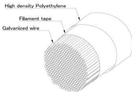
被覆平行線ケーブル (NEW PWS)
